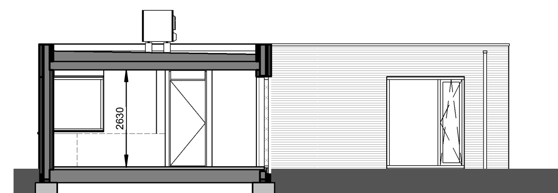
Rechtergevel 1 : 100
