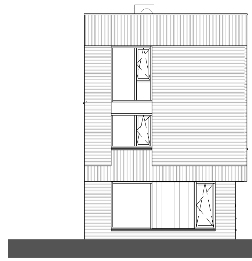
Rechtergevel 1 : 100
