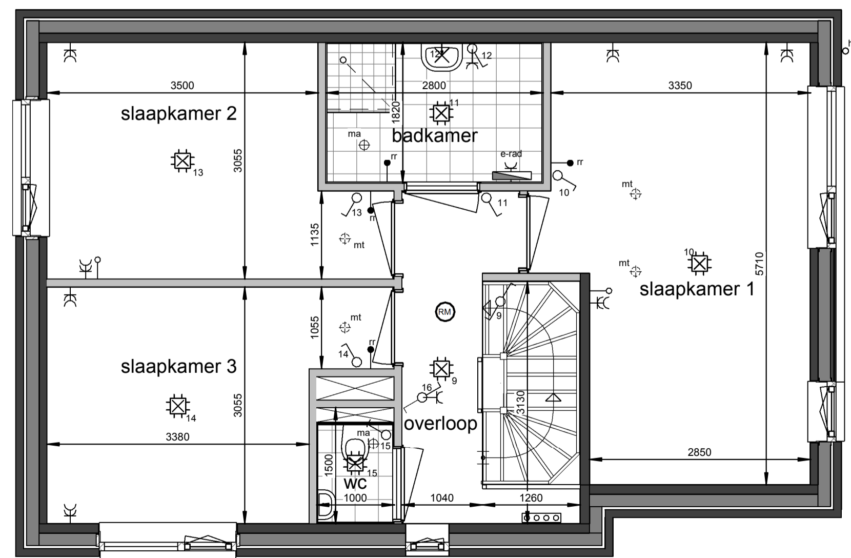
Eerste verdieping 1 : 50
