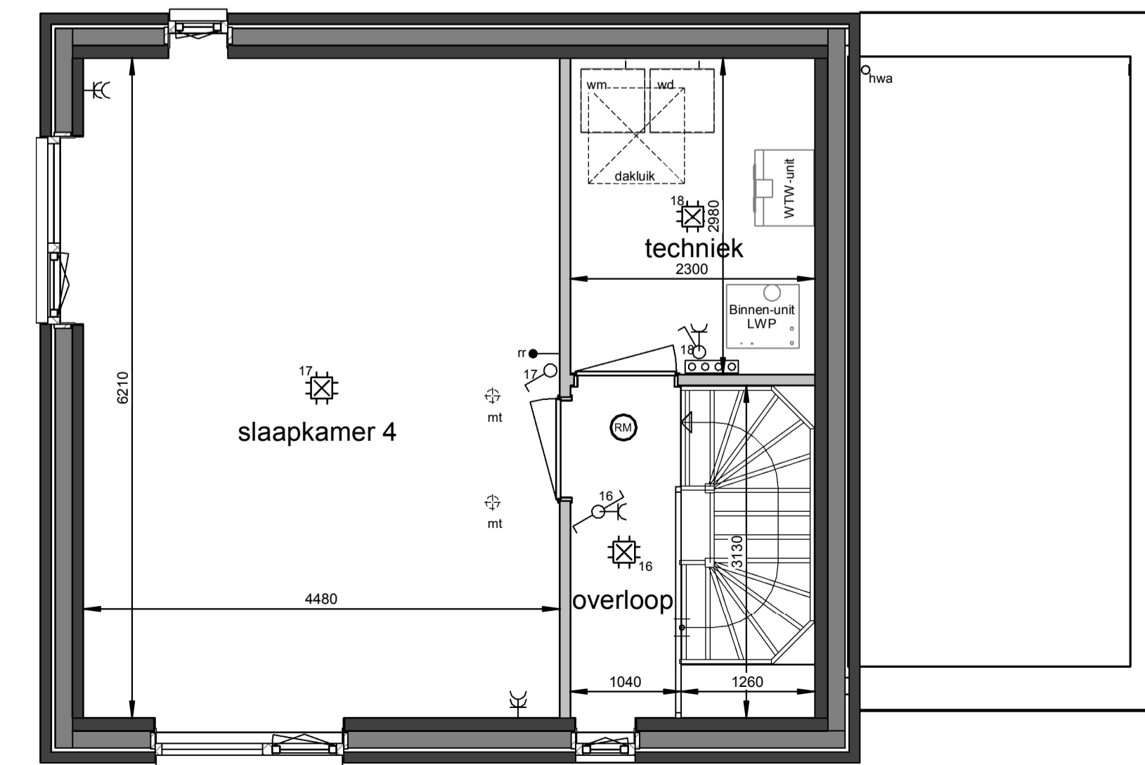
Tweede verdieping 1 : 50
