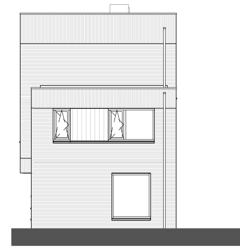
Linkergevel 1 : 100
