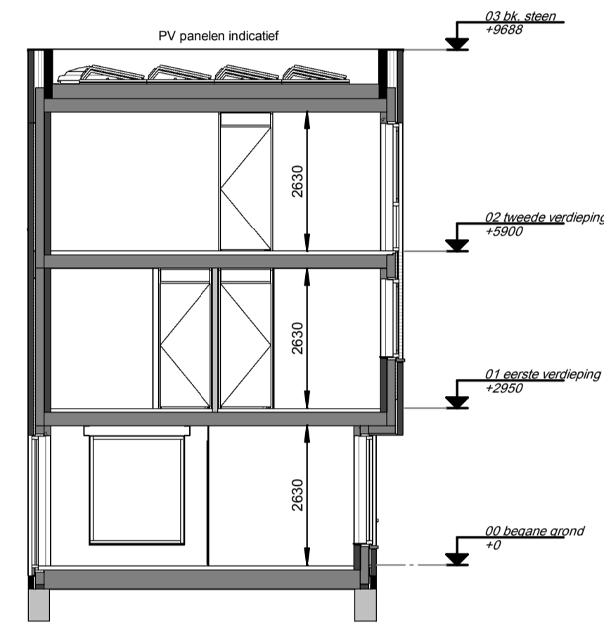
Doorsnede 1 : 100
