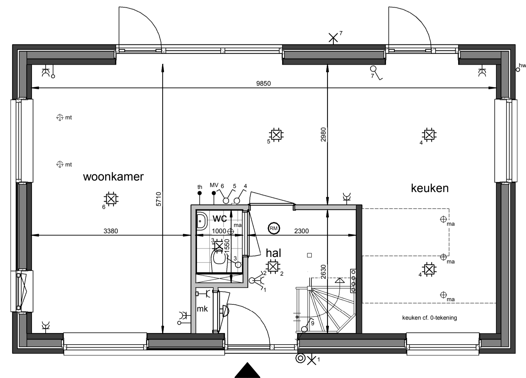
Begane grond 1 : 50
